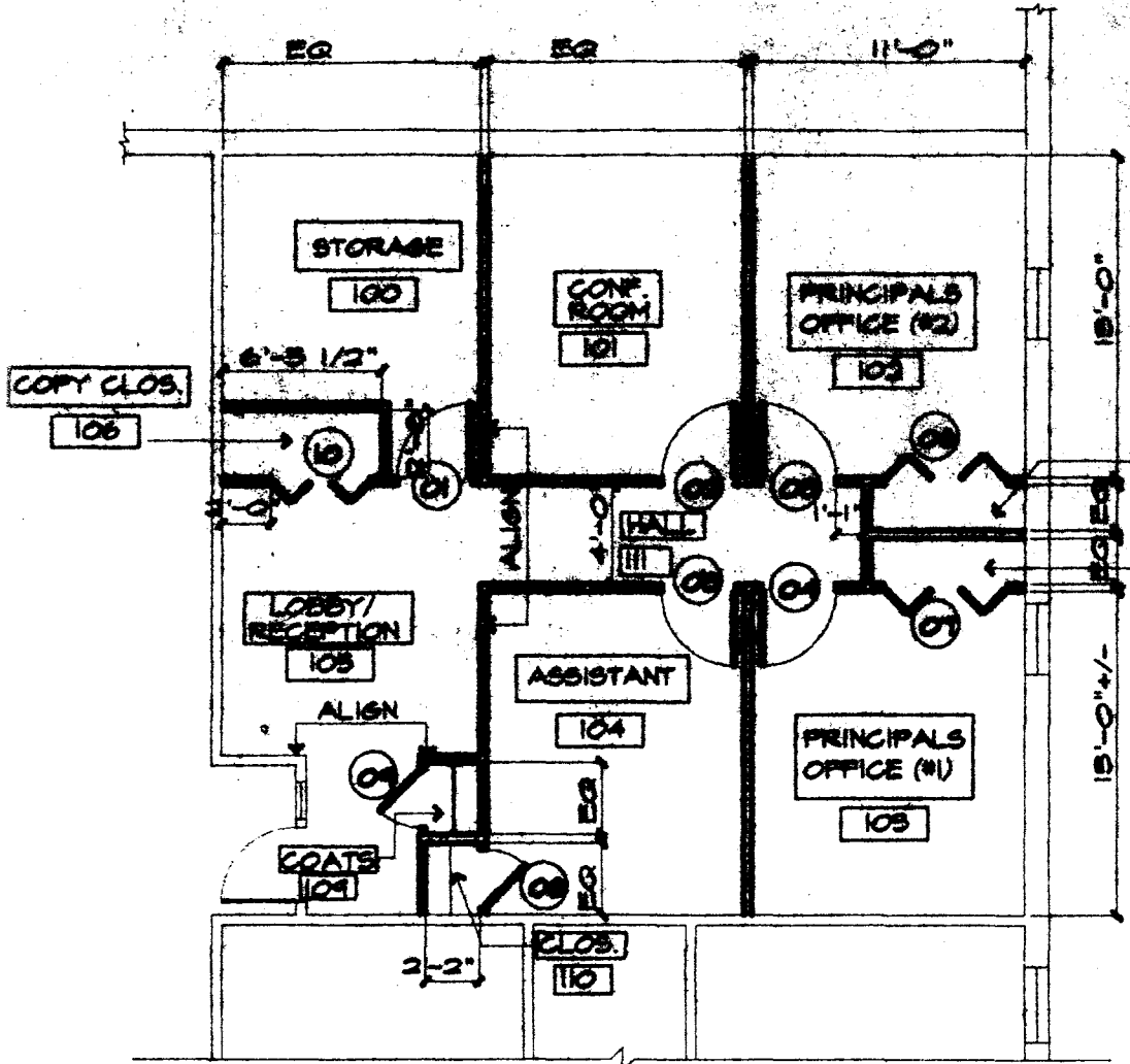
2 TENANT FIT-UP LAYOUT A1 SCALE: 1/8" = 1'-0"
